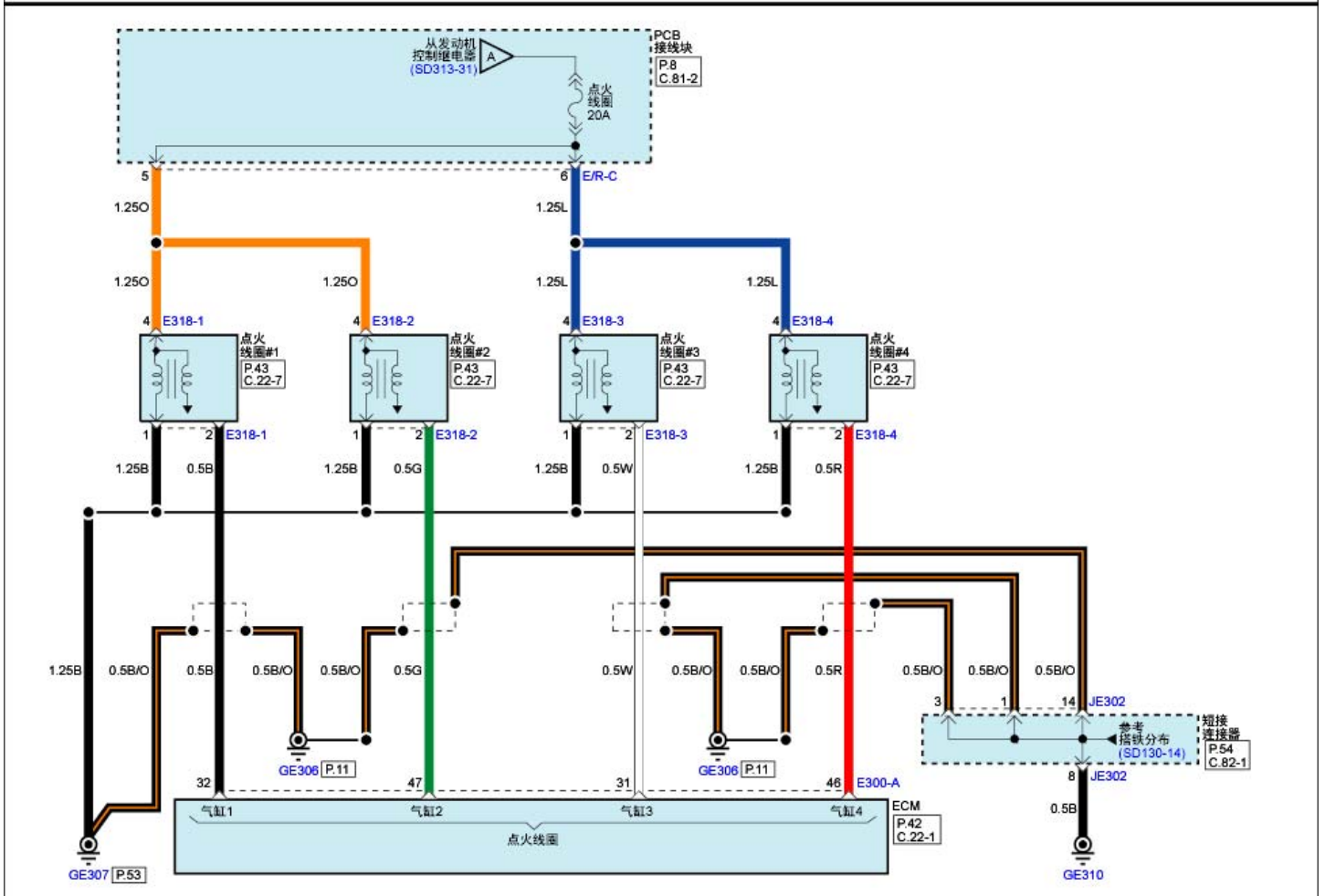
发动机控制系统(G4FJ : GAMMA 1.6L T-GDI)(5)
